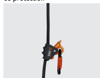
Tendeur en alliage léger muni d'un connecteur
